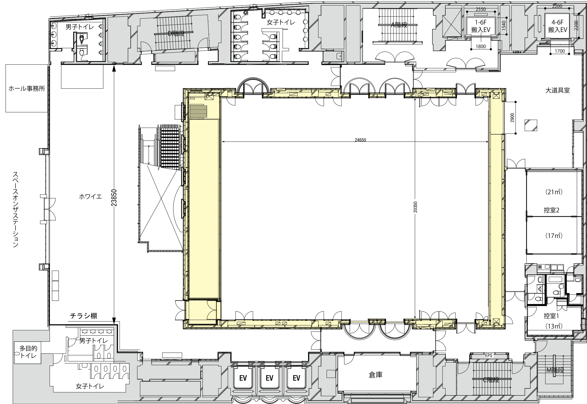
西鉄ホール 平面図
